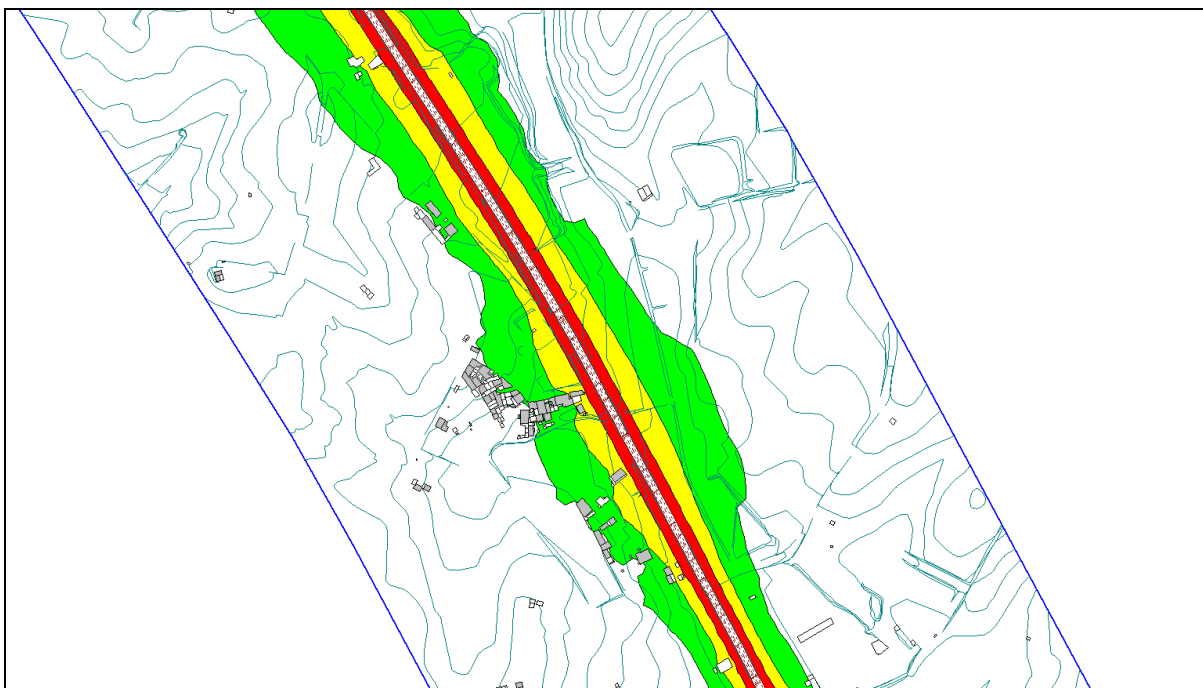
Figura 4.1 – Exemplo de mapa de conflitos para o indicador L_n , que serviu de base para o PA da EN366
